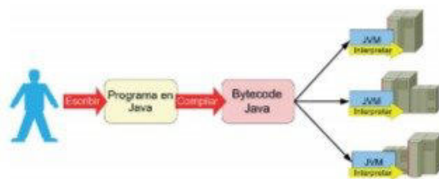
Figura 1.3. Mecanismos de compilación e interpretación para que Java sea un lenguaje multiplataforma y pueda ejecutar el mismo programa en distintos ordenadores instalados con la JVM.
